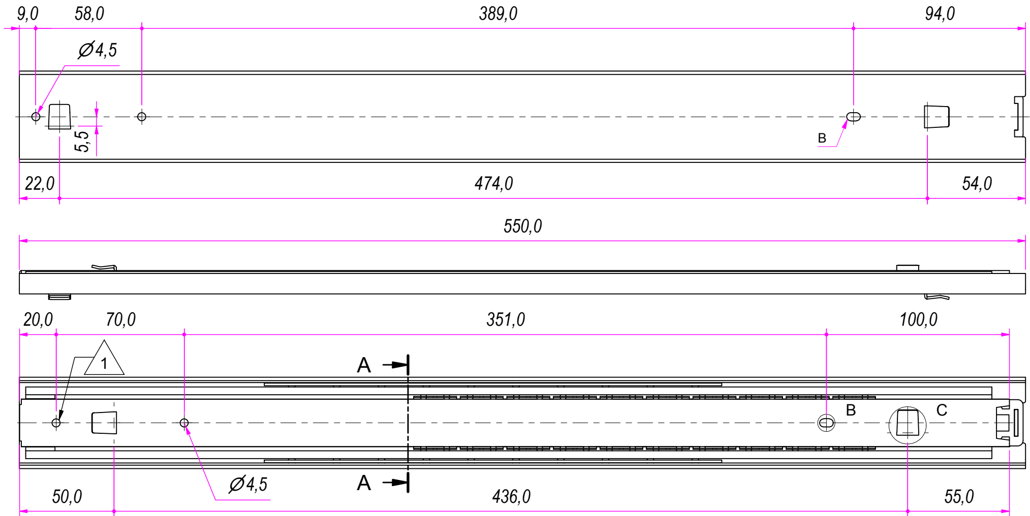
SEZ. A-A
