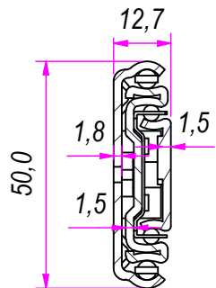
SEZ. A-A
