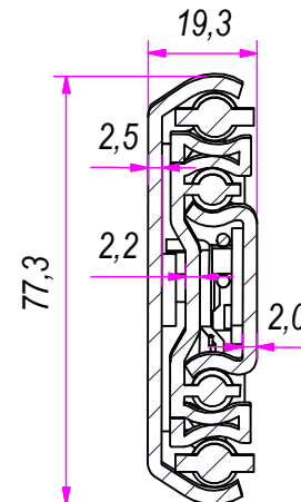
SEZ. A-A
