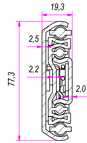
SEZ. A-A
