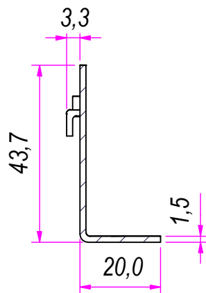
SEZ. A-A
