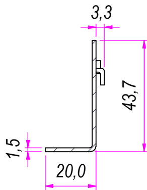
SEZ. A-A
