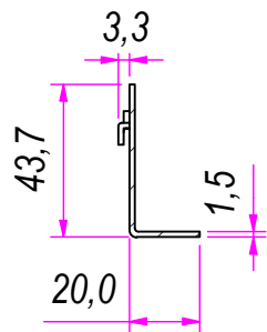
SEZ. A-A
