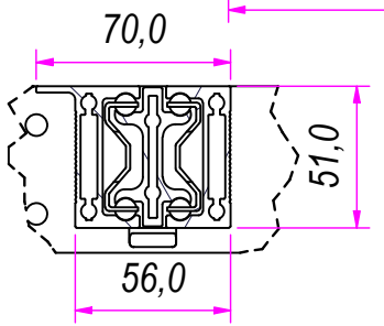
C (1 : 3)
