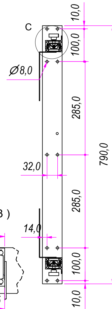
SEZ. A-A
